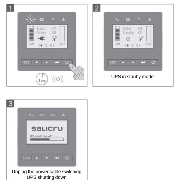
Abb. 28. Herunterfahrsequenz.
