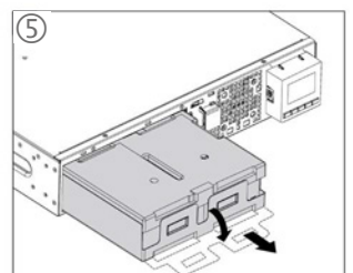
Abb. 39. Schritte zum Entfernen der internen Batterie.
